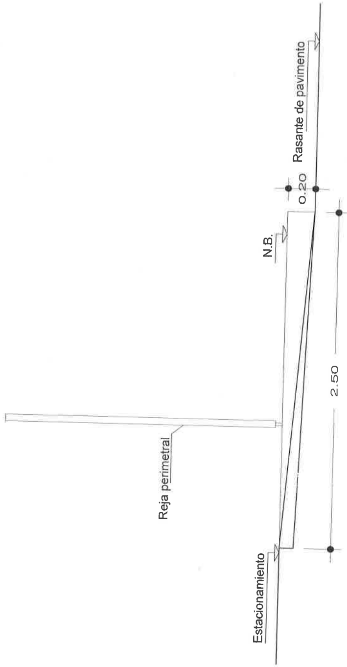
CORTE LONGITUDINAL
